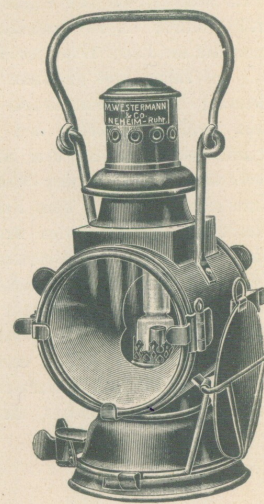
Wärter-Signal-Laterne.
