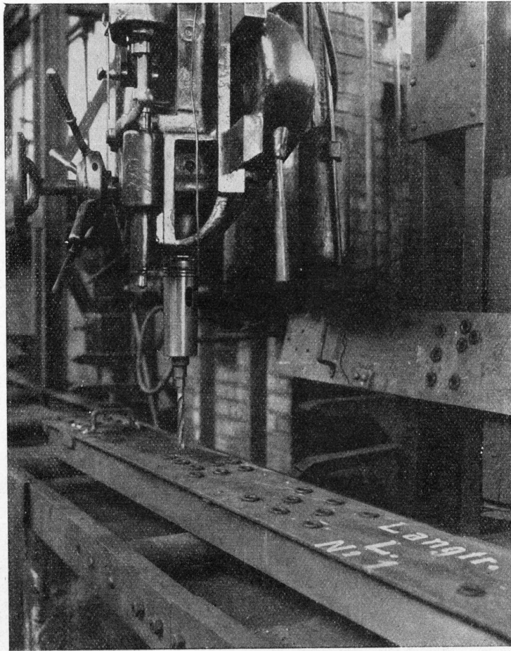
Langträgerbohren
