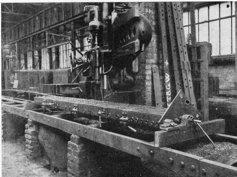
Bohren des Kopfstüdes in dreiseitiger Schablone
