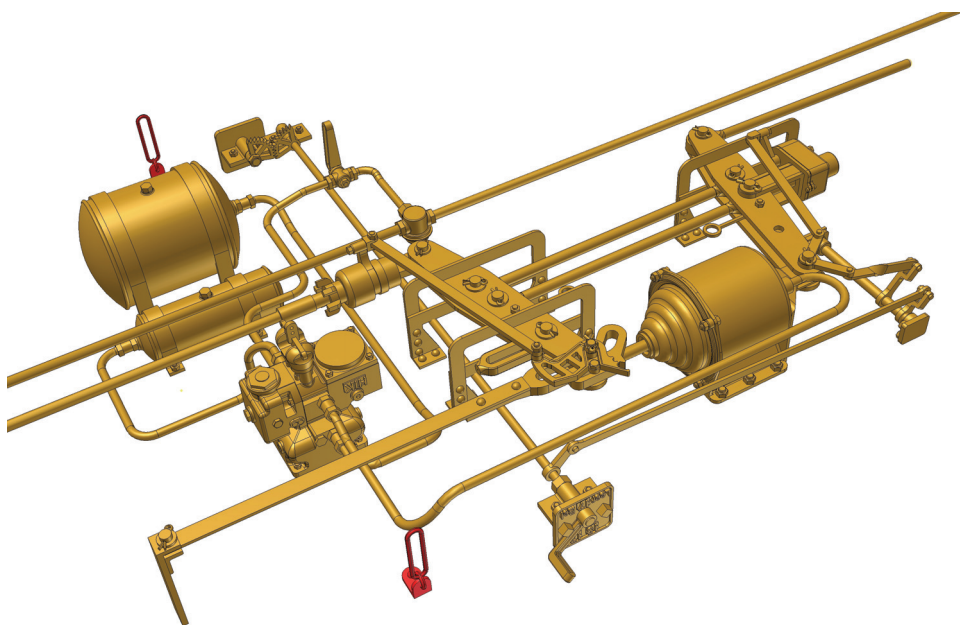
Hildebrand Knorr Bremse für Güterwagen 23
