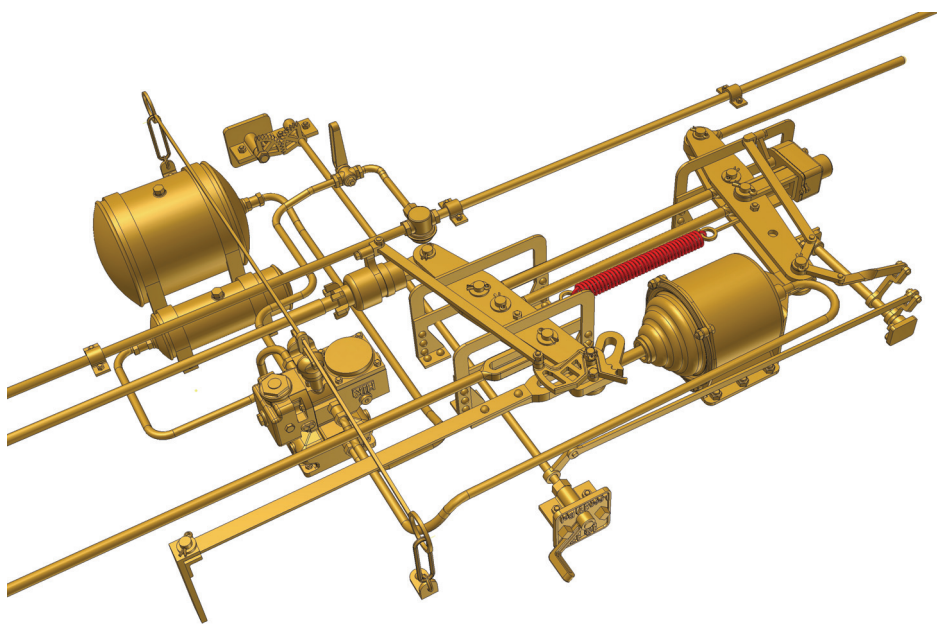
Hildebrand Knorr Bremse für Güterwagen 27
