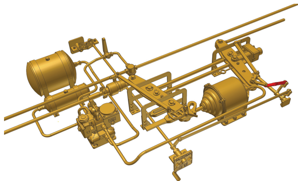
Hildebrand Knorr Bremse für Güterwagen 20
