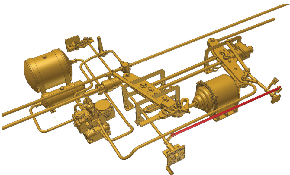
Hildebrand Knorr Bremse für Güterwagen 19
