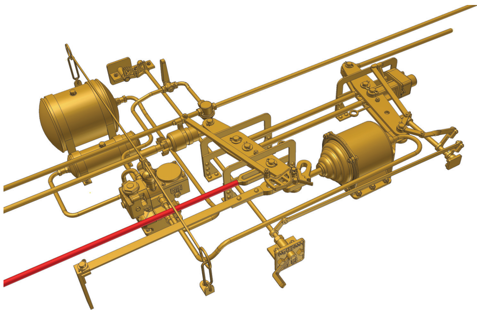
Hildebrand Knorr Bremse für Güterwagen 25
