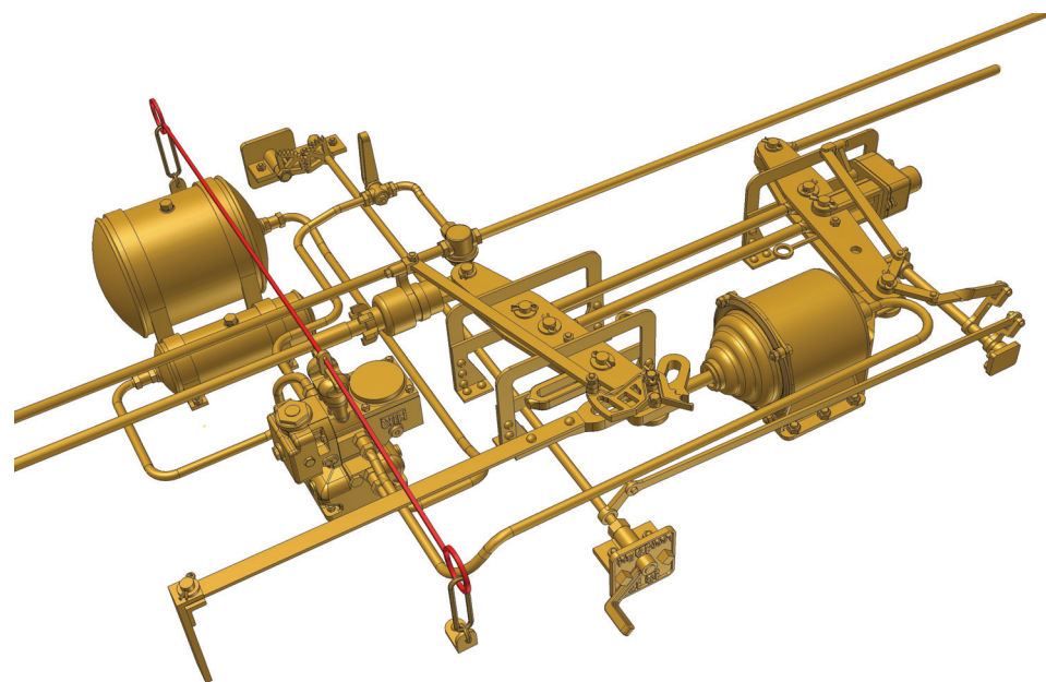
Hildebrand Knorr Bremse für Güterwagen 24
