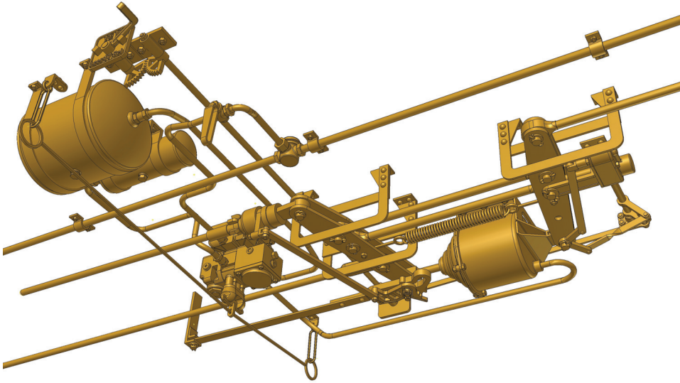
Hildebrand Knorr Bremse für Güterwagen 29
