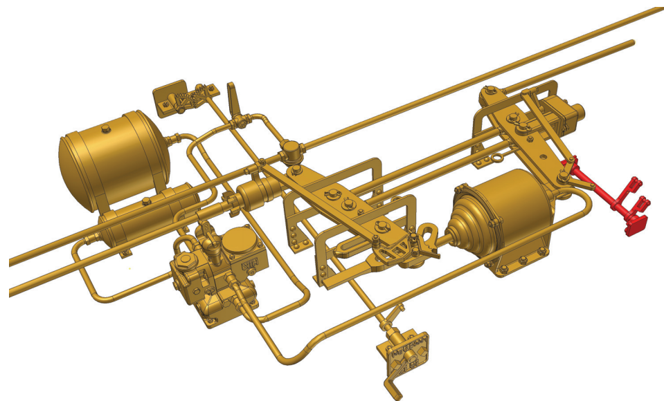
Hildebrand Knorr Bremse für Güterwagen 18
