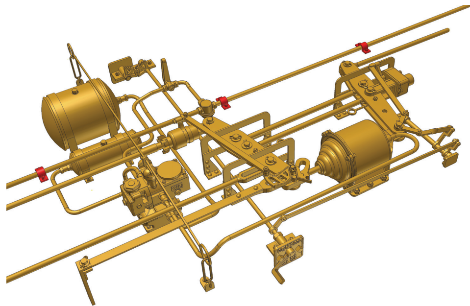
Hildebrand Knorr Bremse für Güterwagen 26
