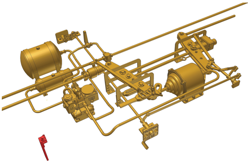
Hildebrand Knorr Bremse für Güterwagen 21
