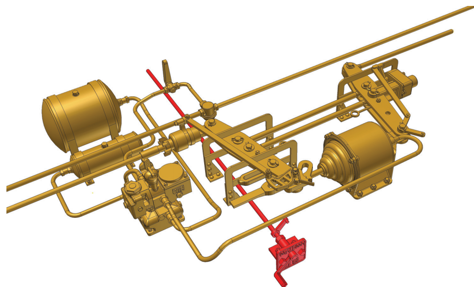
Hildebrand Knorr Bremse für Güterwagen 16
