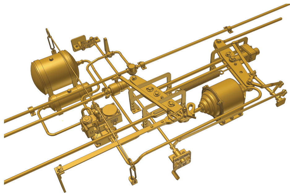
Hildebrand Knorr Bremse für Güterwagen 28
