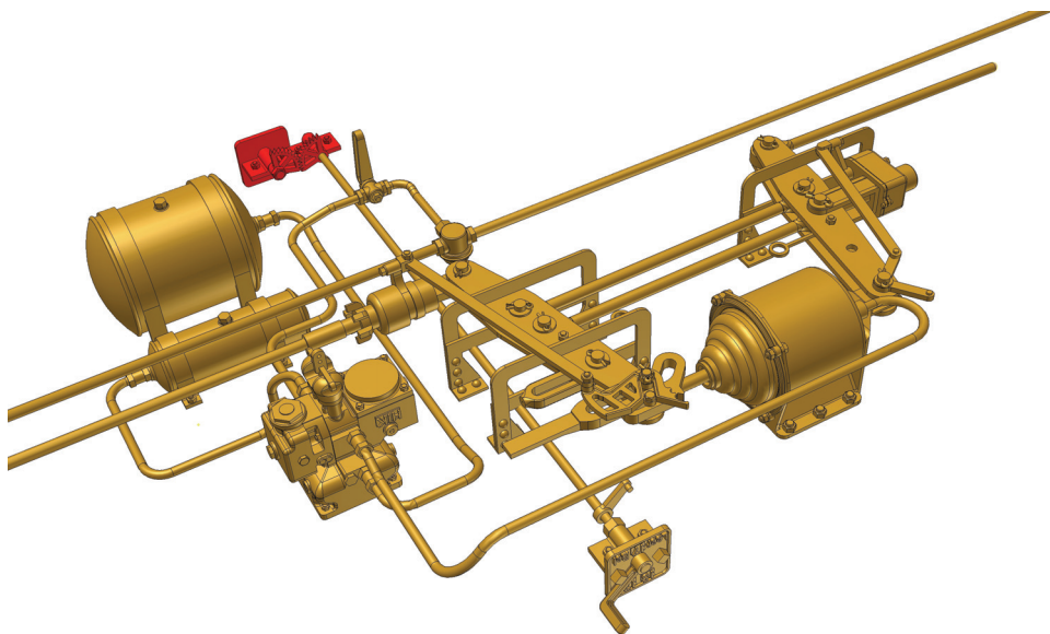
Hildebrand Knorr Bremse für Güterwagen 17
